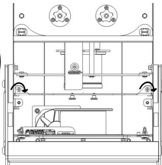
Portagobo con microregolazione messa a fuoco
