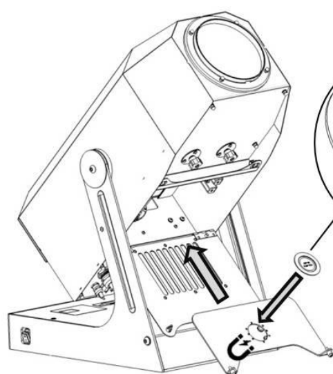
Portagobo con microregolazione messa a fuoco
