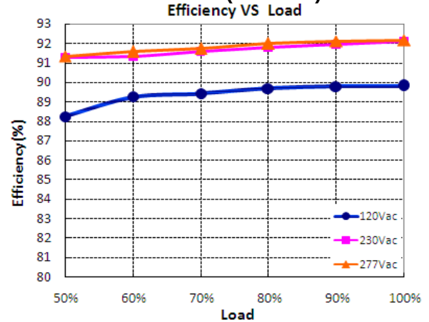
X6-105Y150 (Io=1.05A)
