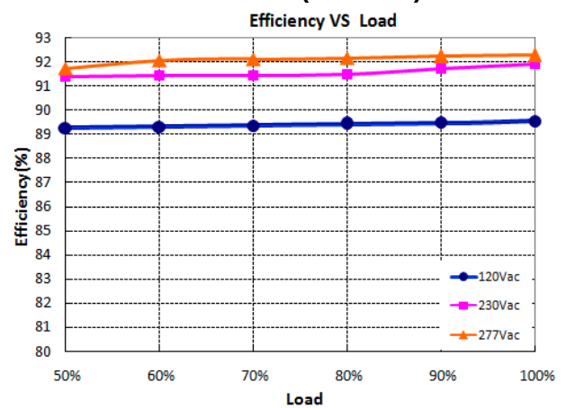
X6-105Y150 (Io=1.05A)
