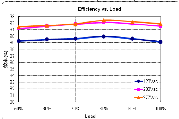
X6-105Y062 (Io=1.69A)
